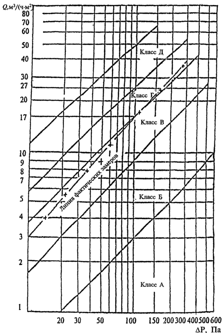
Рисунок Б.1. Пример определения класса воздухопроницаемости
